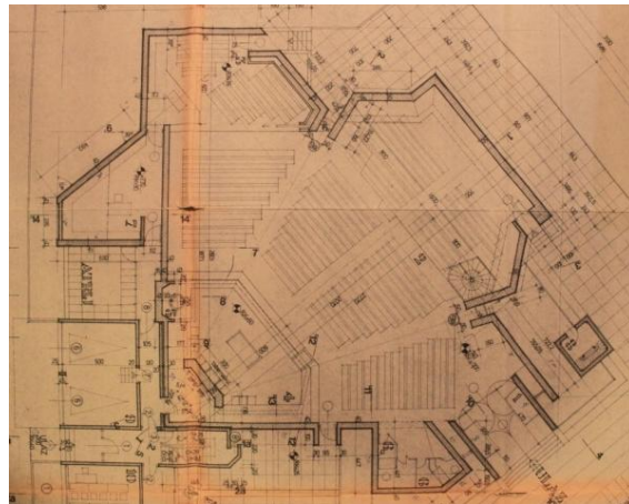
Sl. 112. Crkve Bezgrešnog začeća BDM, Zadar, tlocrt Izvor: Arhiv Župe Bezgrešnog začeća BDM - Zadar
