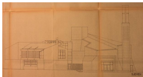
Sl. 114. Crkva Uznesenja BDM, Zadar, zapadna fasada Izvor: Arhiv Župe Bezgrešnog začeća BDM - Zadar
